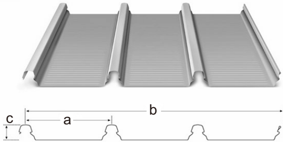
kliplok 406/700
