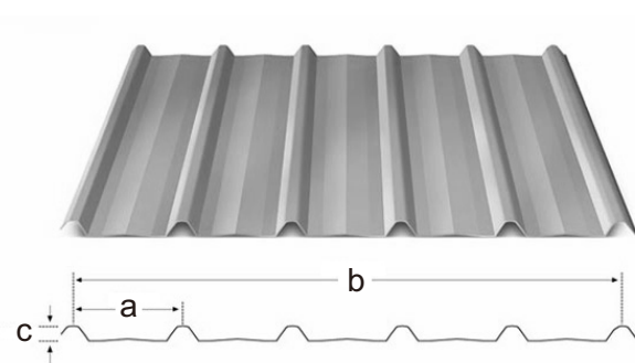
trimdek
