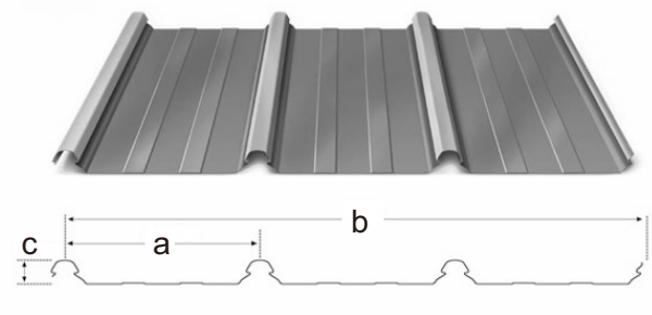
kliplok 770
